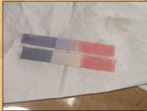
Roccella montagnei
